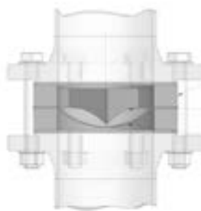
Gehäuse Dreiteil-Messer Umkehr-Berstscheibe
